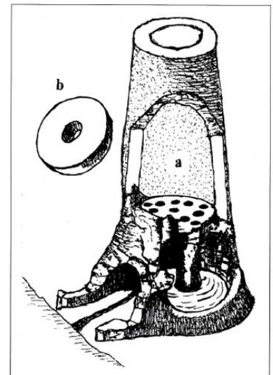
Fig. 7a - Forno etrusco a doppia camera con setto forato. Fig. 7b - "Ciambella" di ferro ottenuta. Fig. 7a - Double chamber etruscan furnace with perforated plate. Fig. 7b - Iron "ring" obtained.
