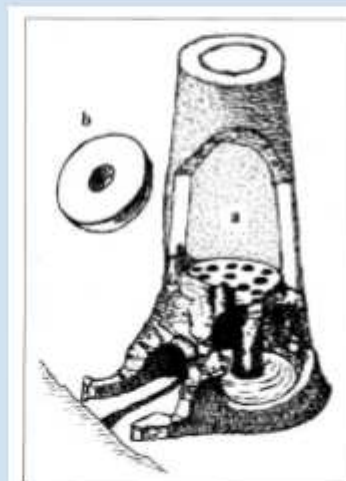
Fig. 74 - Forno etrusco a doppia camera con alto forno. Fig. 75 - "Candelina" di ferro etrusco. Fig. 76 - Double chamber etruscan furnace with perforated plate. Fig. 77 - Iron "ring" etruscan.
